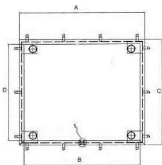
Grubenrahmen
